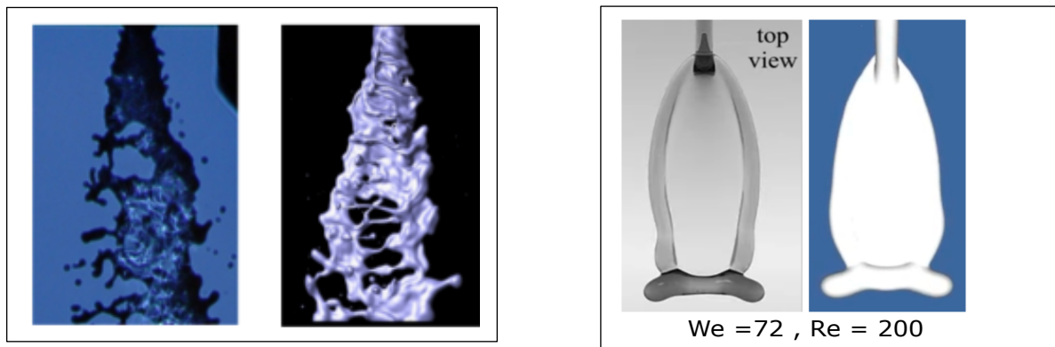
Fig 2 : Comparaison exp./num. : injecteur triple disque (à gauche) [8], impact de jets (à droite)
