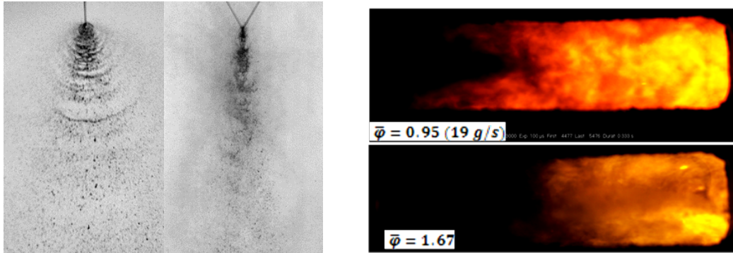
Fig 1 : Pulvérisation par impact de jets et visualisation de la combustion stabilisée
